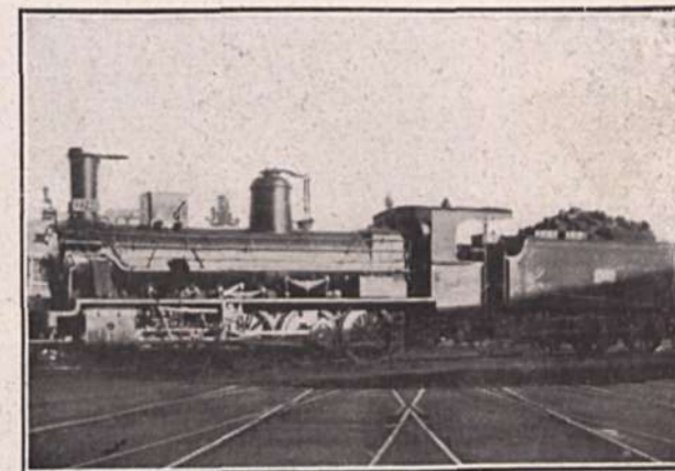
Tipo de las nuevas locomotoras adquiridas por la Compañía de ferrocarriles del Norte FOTS. A. RIVAS
