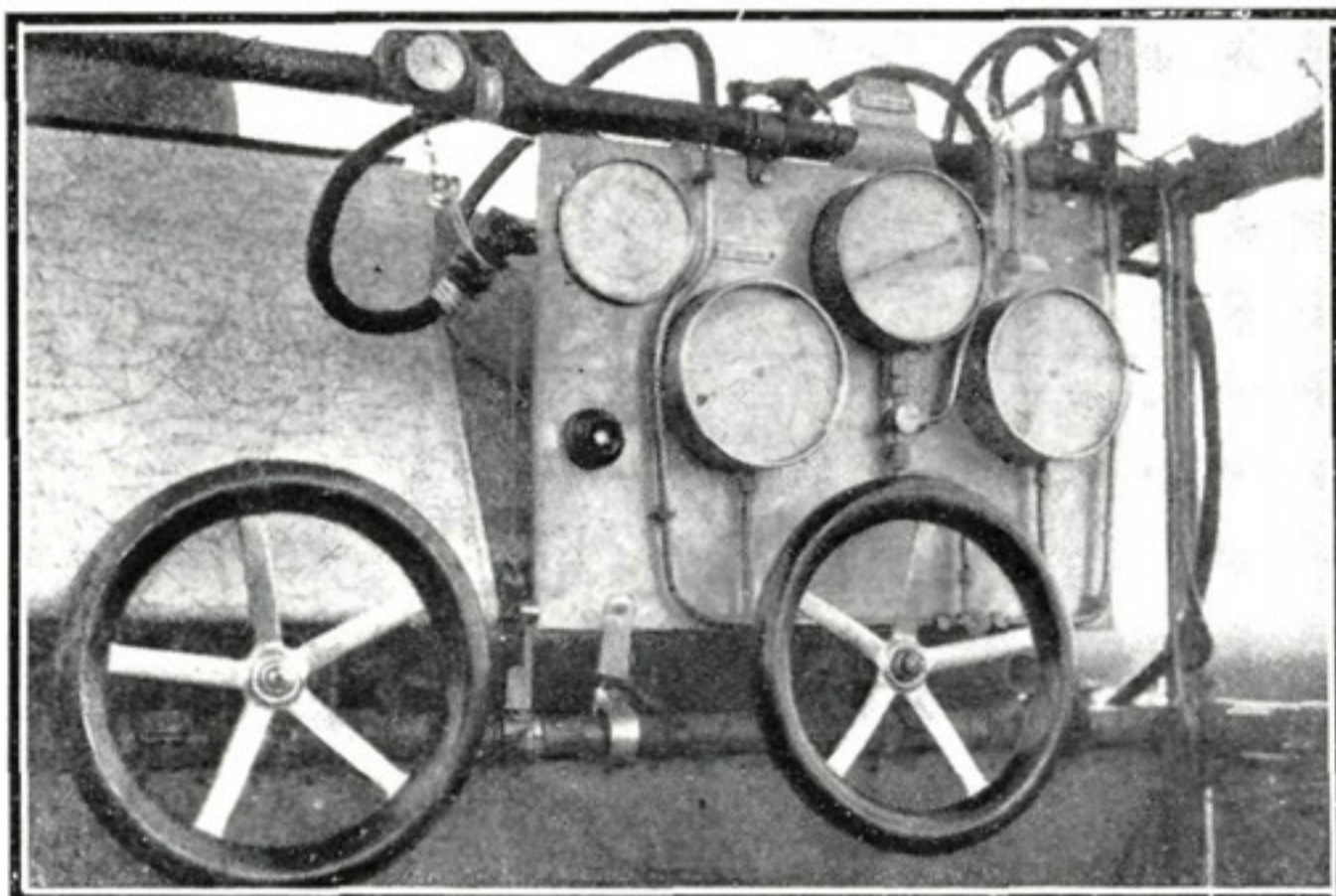
Los volantes y manómetros de dirección que maneja el comandante del dirigible
